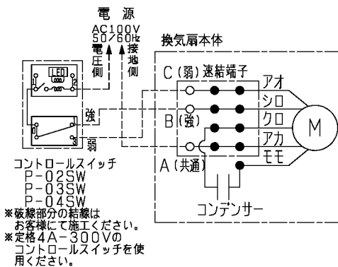
■ 結線図
