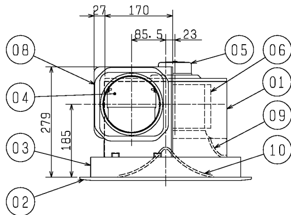
■ 天吊金具（同梱）取付位置（4点吊り）
