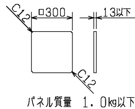
■ パネル寸法
